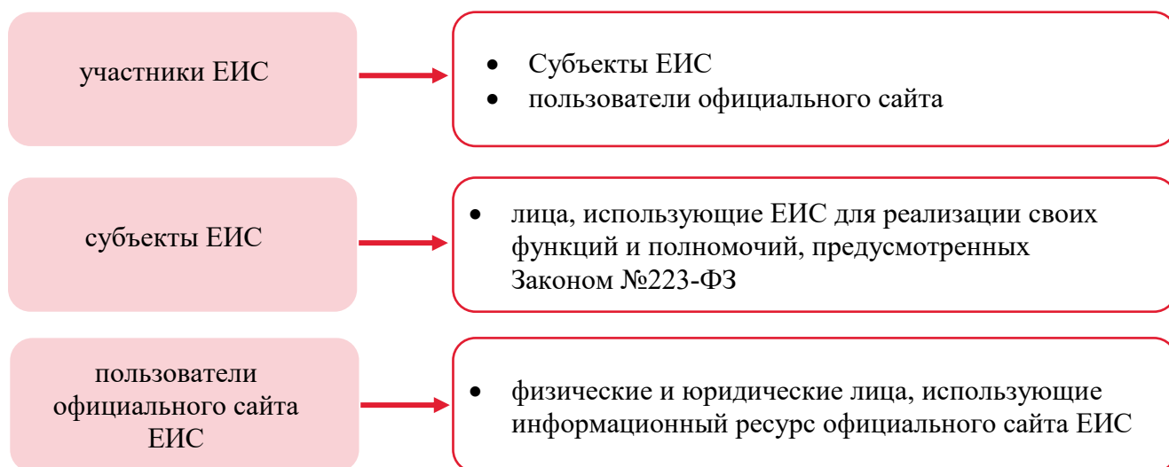
Рис. 2. Терминология ЕИС
