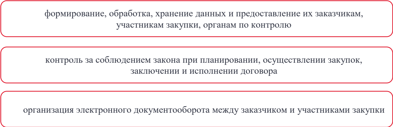
Рис. 1. Функции ЕИС
